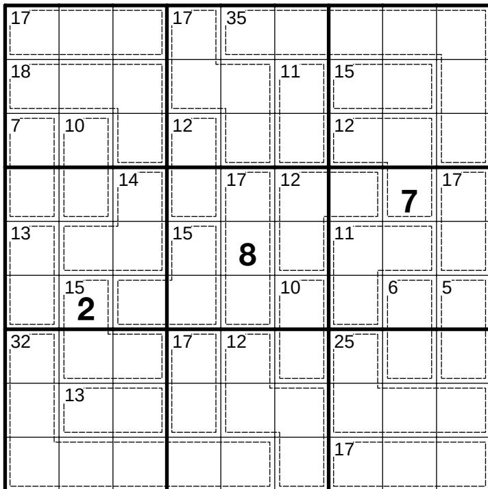
Killer Sudoku #663
