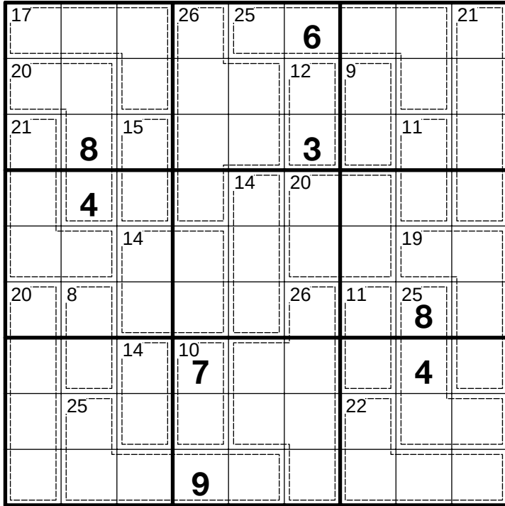
Killer Sudoku #661
