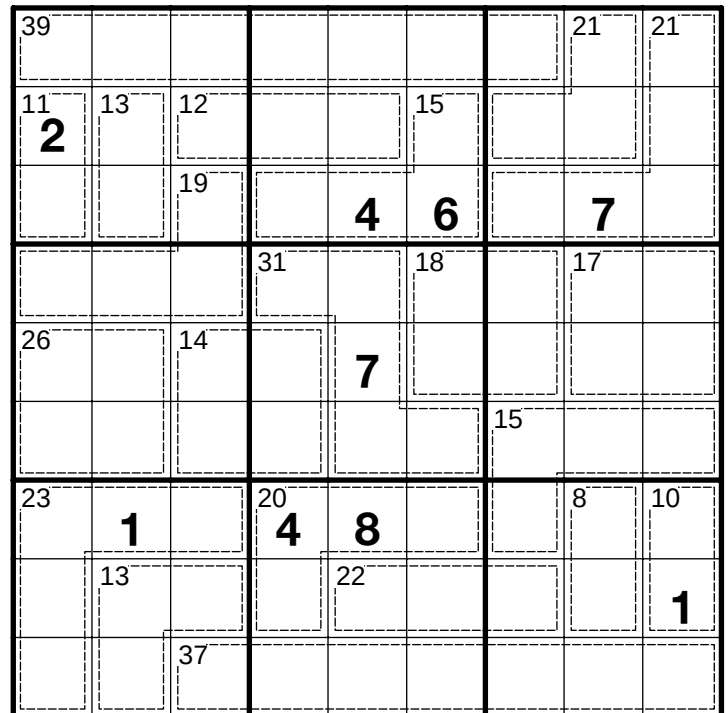
Killer Sudoku #664
