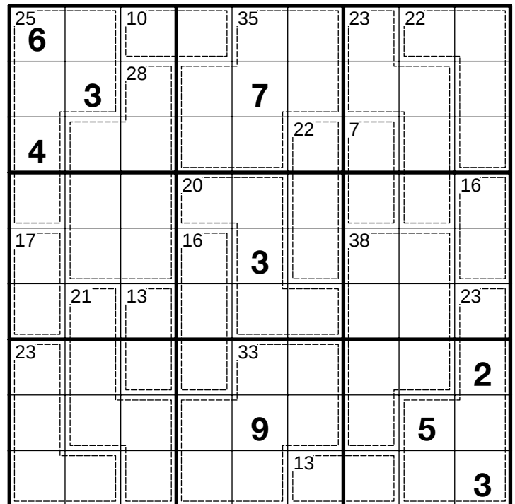
Killer Sudoku #716
