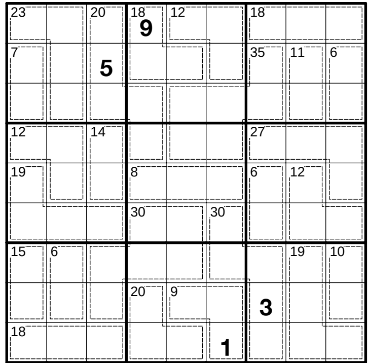
Killer Sudoku #714
