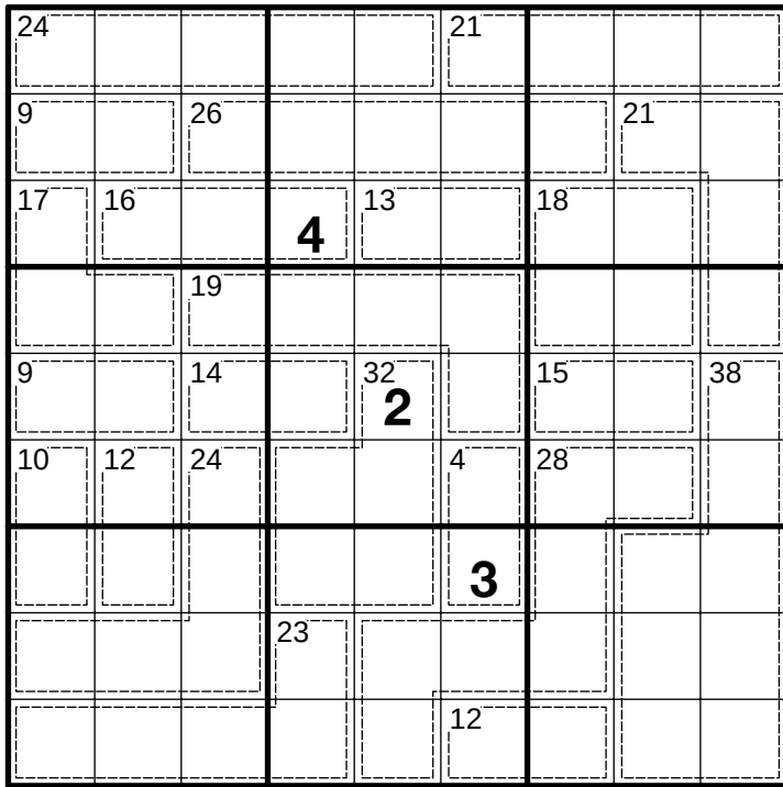
Killer Sudoku #713
